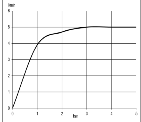
Durchflussdiagramm
